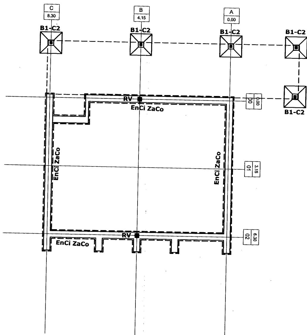
PLANO ESTRUCTURA ESC. 1:100
