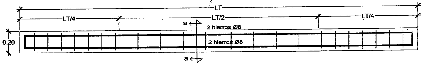
DETALLE 02 ESC. 1:20
