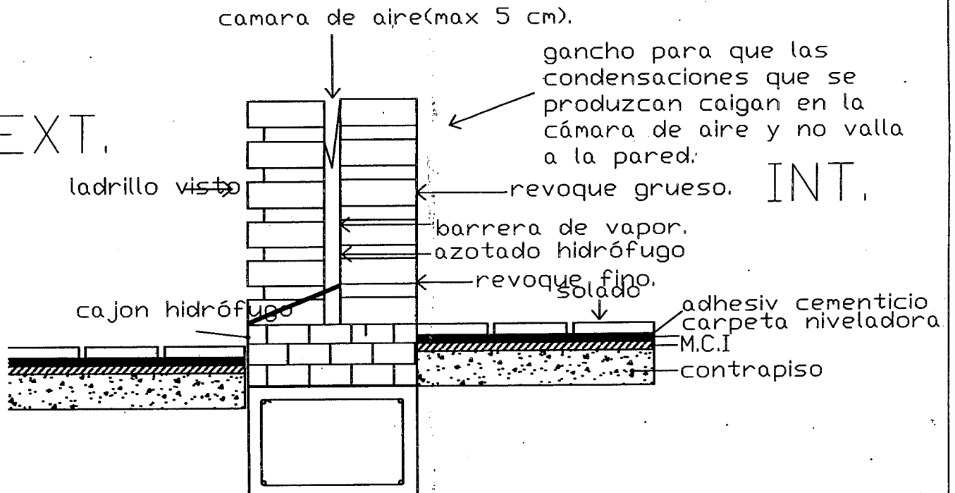
DETALLE 01 ESC. 1:20
